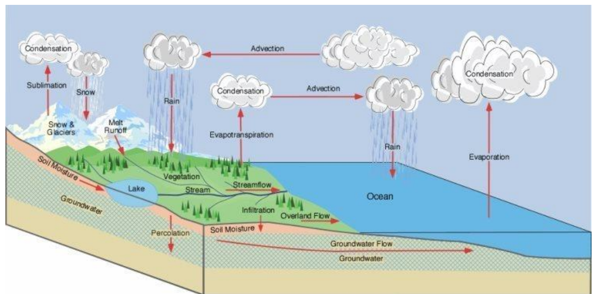
Siklus air dan proses terjadinya hujan. Sumber gambar: physicalgeography.net
